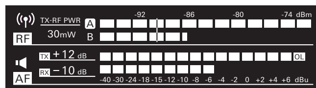
Écran de mesure de niveau
