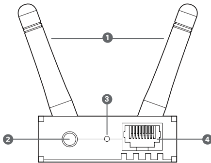
Abbildung E – Unterseite ATW-RU13
