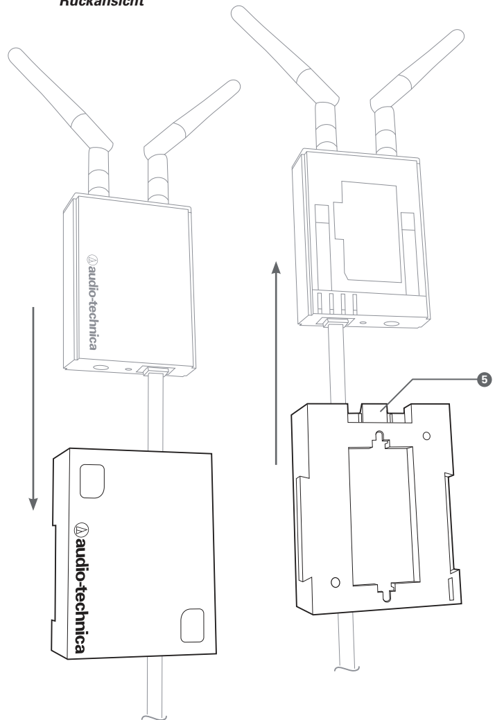
Abbildung F – AT8690 RU13 Halterung Vorder- und Rückansicht
