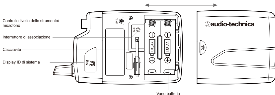
Figura D — Trasmettitore UniPak® ATW-T1001EX
