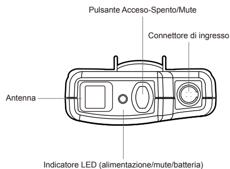
Figura E— Trasmettitore UniPak®
