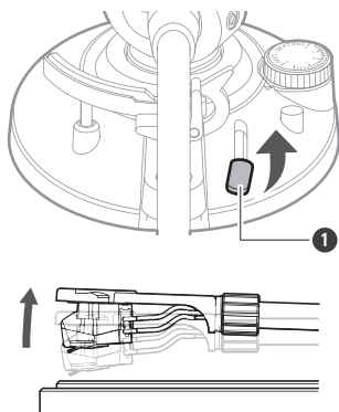
1 Bedieningshendel voor toonarmlift
