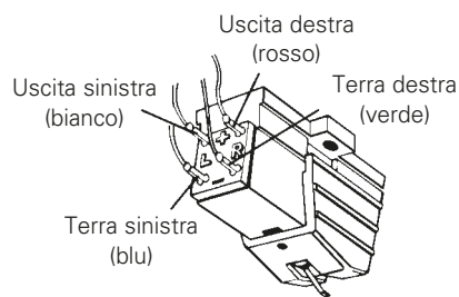
Figura 8 – Collegamenti elettrici
